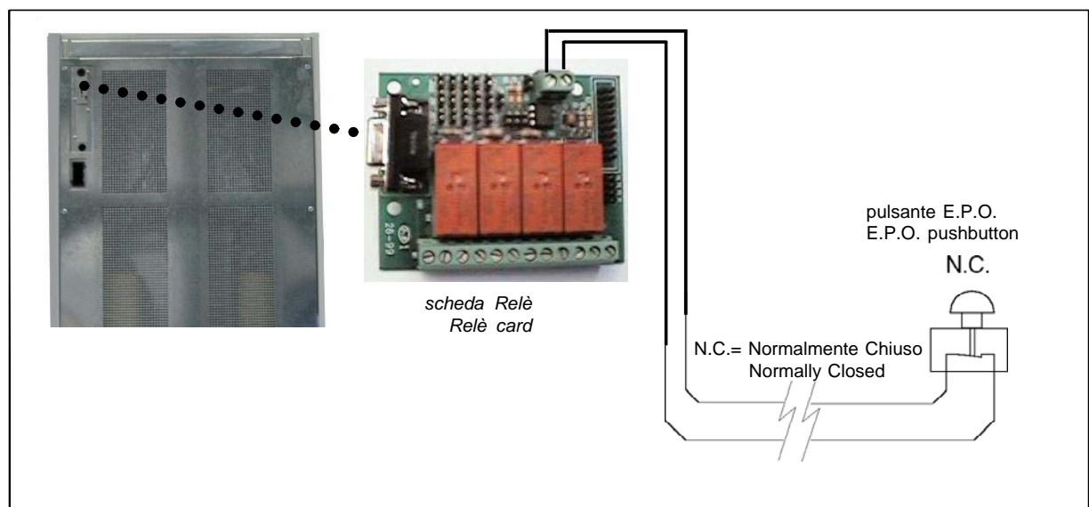
Fig. 2.5 - Collegamento del pulsante E.P.O. - E.P.O. connection
