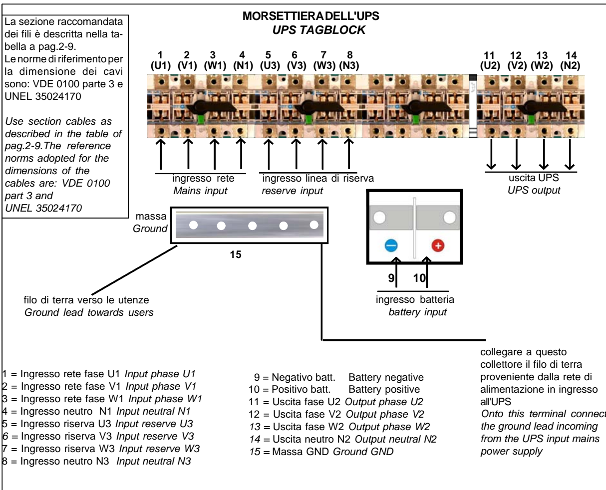
Fig. 2.3 - Collegamenti alla morsettiera dell'UPS Wiring on the UPS tagblock
